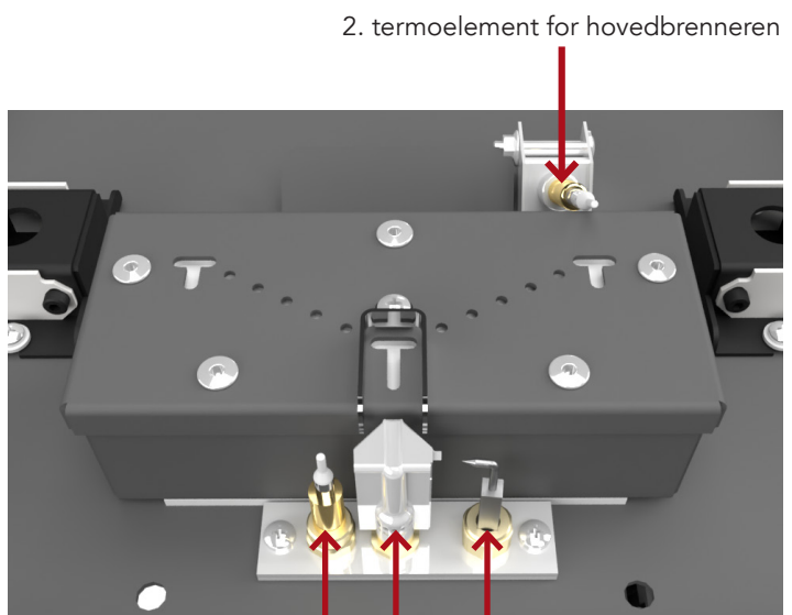
1. termoelement
