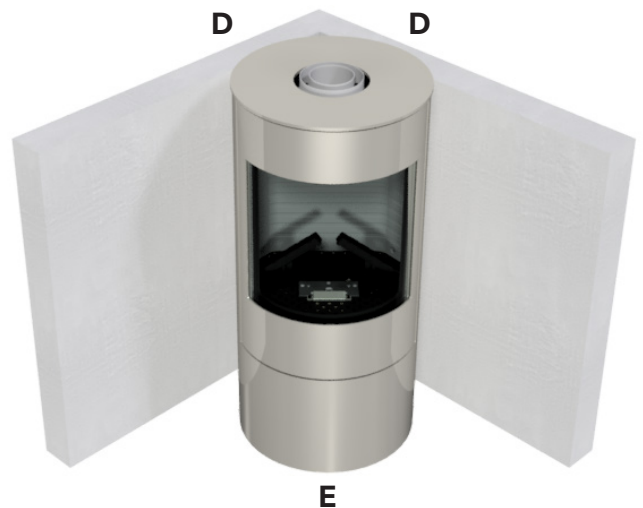
Installatie in een hoek
