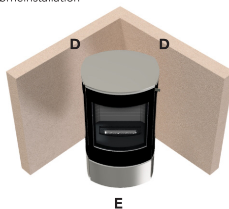
Hjørneinstallation
